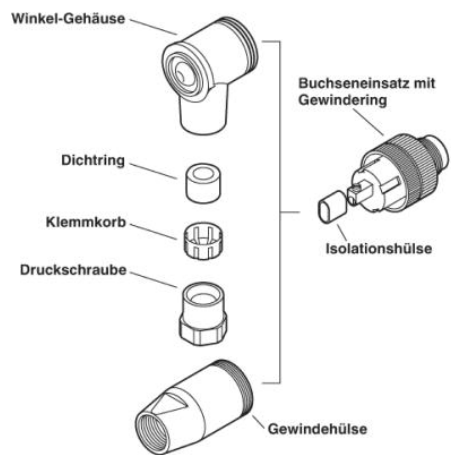
Stecker/Buchse M12
