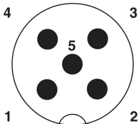
Stecker/Buchse M12
