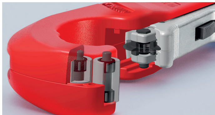
Krążek tnący i cztery rolki prowadzące pracują praktycznie bez tarcia podczas cięcia dzięki wysokiej jakości łożyskom igielkowym - wyjątkowo łatwe cięcie rur ze stali nierdzewnej
