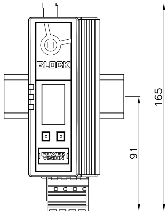
Darstellung mit Anschlußklemmen
