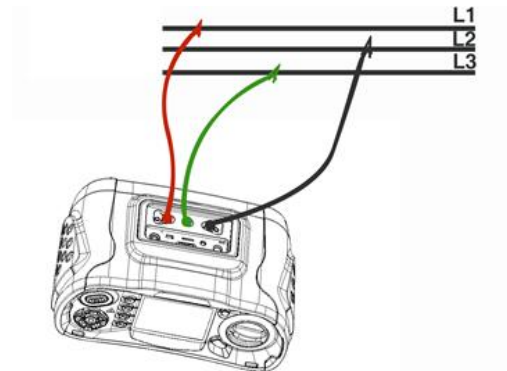
Anschluss der Phasensequenzmessung
