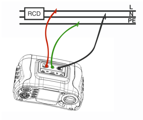
Anschluss bei der FI Messung
