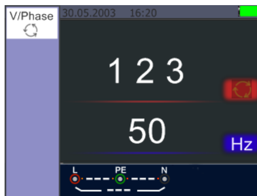
Richtige Phasensequenz L1, L2, L3
