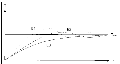
Abbildung 5: Regelverhalten der einzelnen Energie-Werte (schematisch)
