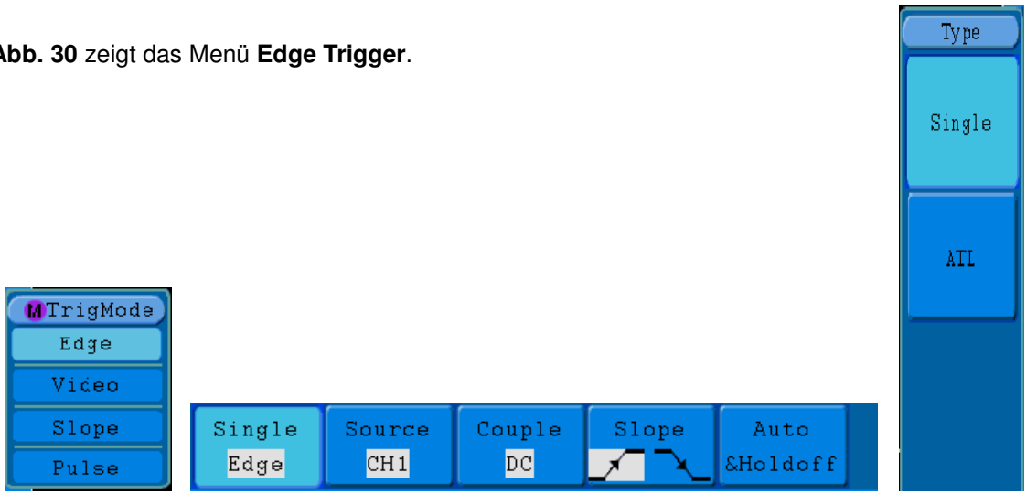
Abb. 30 Edge-Triggermenü
