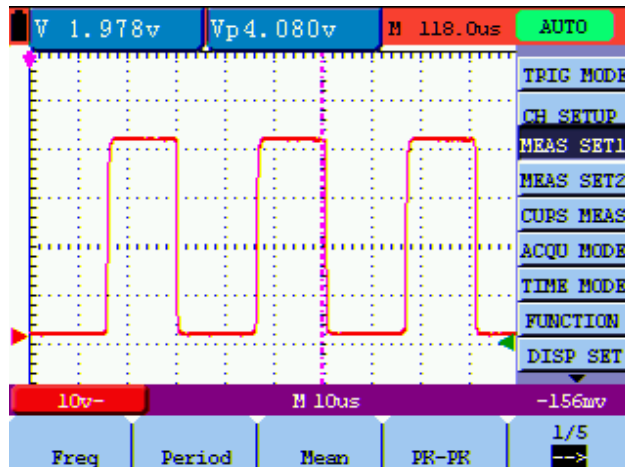
Abbildung 11: automatische Oszilloskop-Messungen
