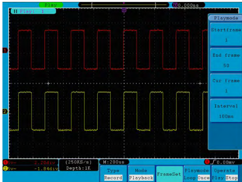
Abb. 50 Wellenform-Wiedergabe
