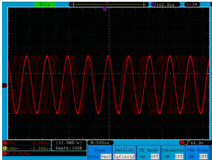
Abb. 44 Unendliche Nachleuchtzeit
