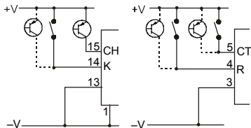
Source (PNP) Inputs
