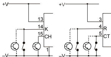
Sink (NPN) Inputs
