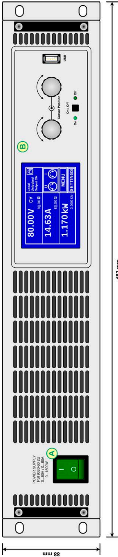
Bild 1 - Vorderseite
