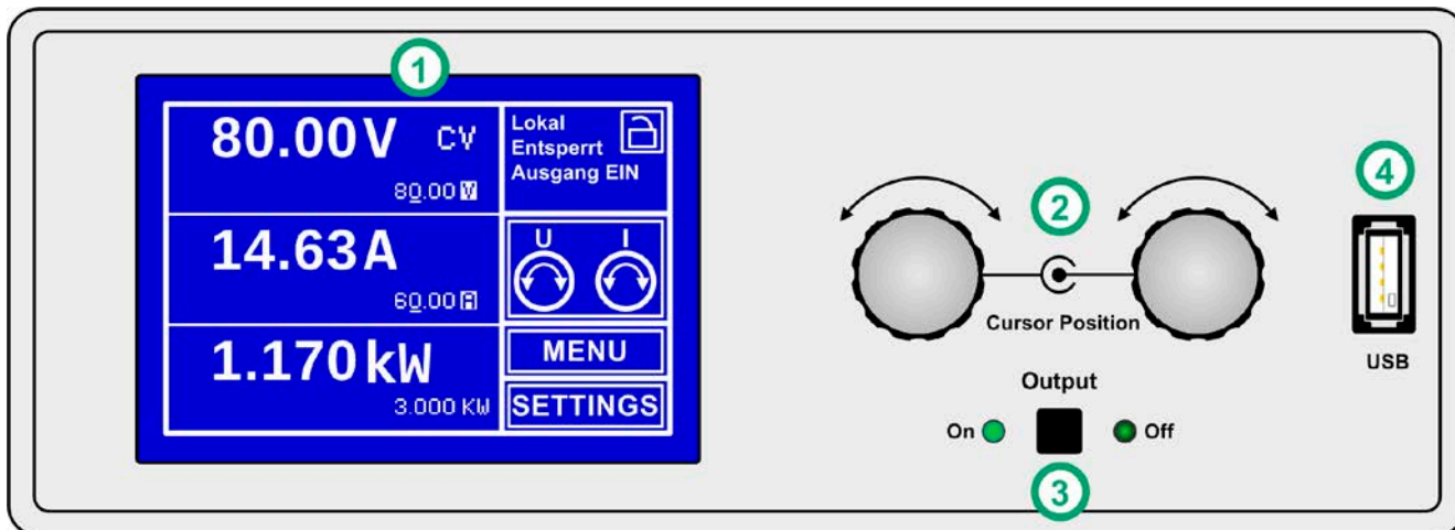
Bild 6 - Bedienfeld
