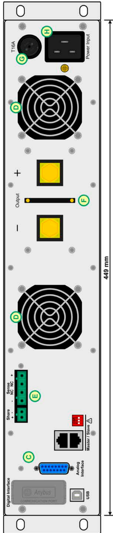
Bild 2 - Rückseite
