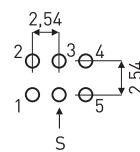
Pin out Mini USB
