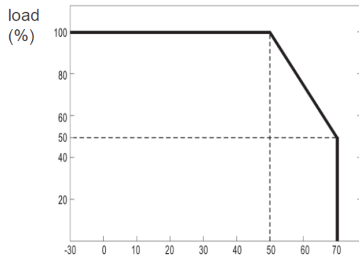
Environment temperature(°C)
