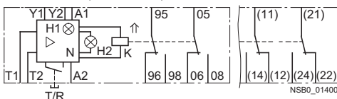
3RN10 13-...0 (monostable)
