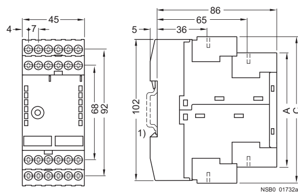
3RN10 62
