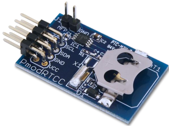
The PmodRTCC.
