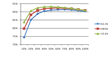
RSD-300C-48
