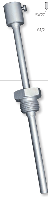
TH08/xx/90 Edelstahлтаuchhülse mit Halsrohr Stainless steel immersion sleeve with neck tube doigt de gant en acier inox avec tube prolongateur Гильза погружная из высококачественной стали с горловиной
