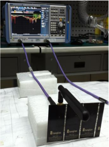
Antenna bent
