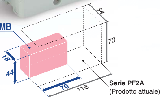
Confronto con PFMB7201 e PF2A721-03
