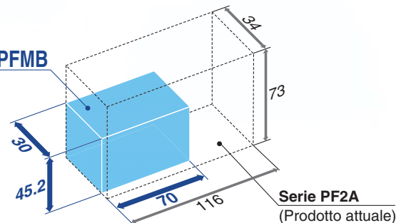
Confronto con PFMB7501-04 e PF2A751-04
