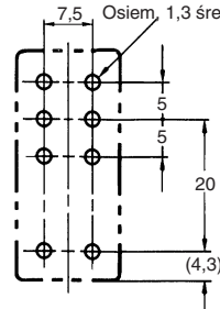
Otworki montażowe
